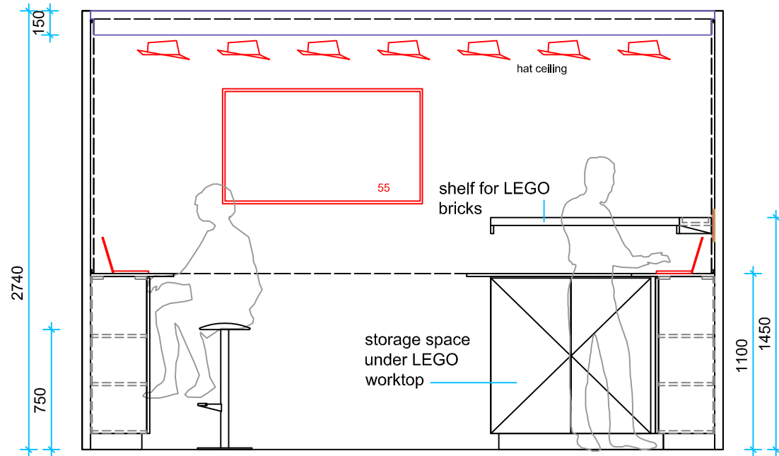
vooraanzicht
