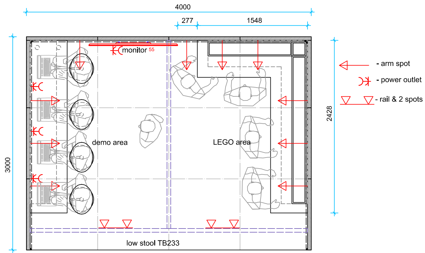
bovenaanzicht
